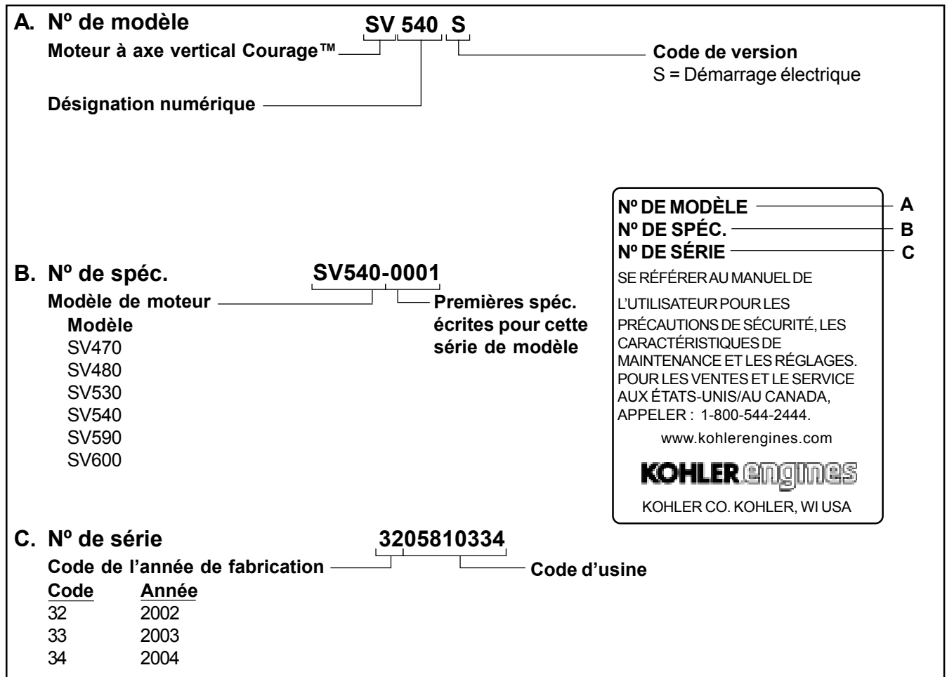
Figure 1-2. Explication des numéros d'identification du moteur.
