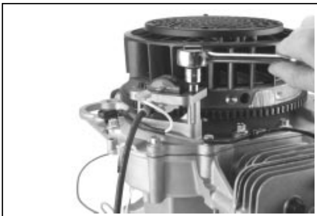
Figure 8-21. Dépose du module d'allumage.
