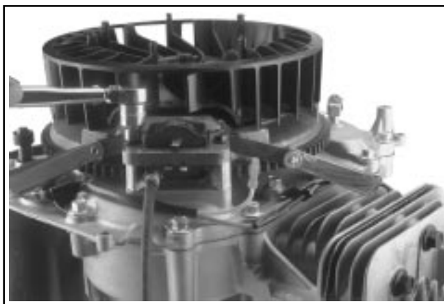
Figure 10-49. Réglage de l'intervalle.
