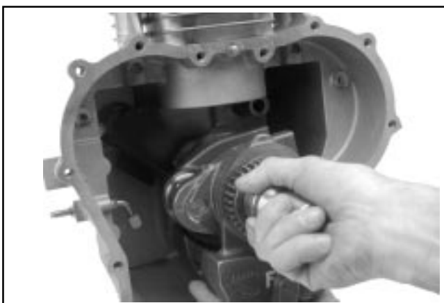
Figure 8-48. Dépose du vilebrequin et des masses d'équilibrage.
