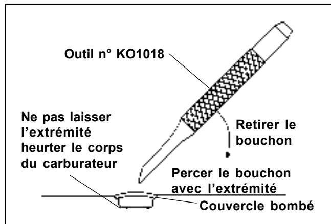
Figure 5-6. Dépose du couvercle bombé.
