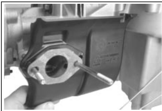
Figure 8-19. Dépose du déflecteur thermique.
