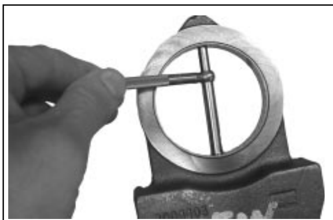
Figure 9-4. Mesure de la surface de support de la masselotte.
