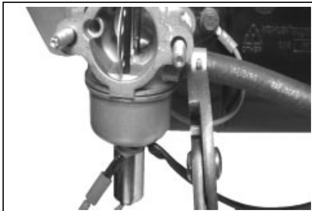
Figure 8-11. Débranchement de la canalisation du carburant du carburateur.
