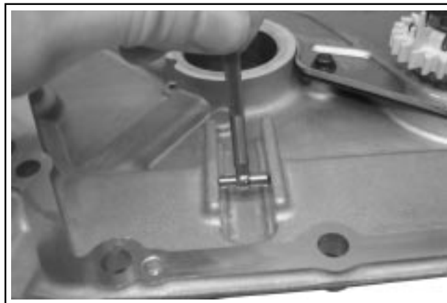
Figure 9-7. Mesure de la largeur du canal de guidage de la plaque de fermeture.
