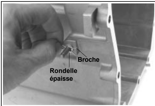
Figure 10-4. Fixation de l'arbre du régulateur.
