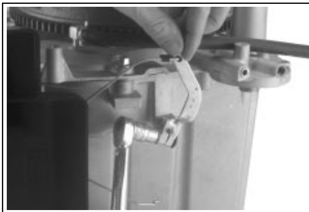
Figure 5-22. Serrage de l'écrou du levier du régulateur.
