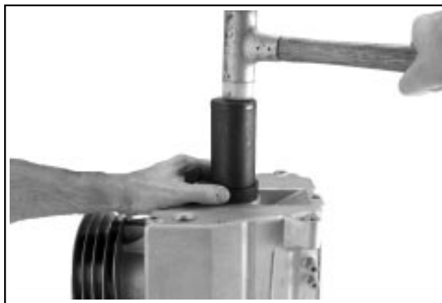
Figure 10-1. Installation du joint d'huile côté transmission.
